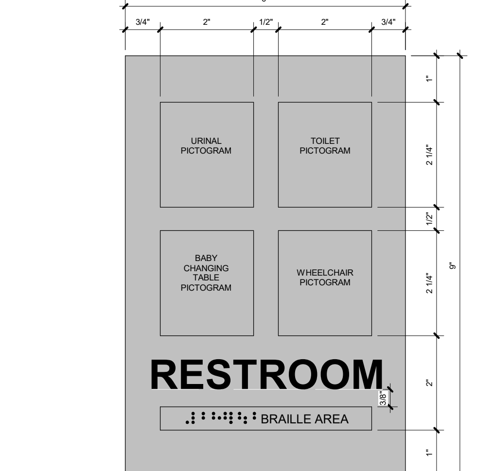
S-2A SCALE: 6" = 1'-0"
