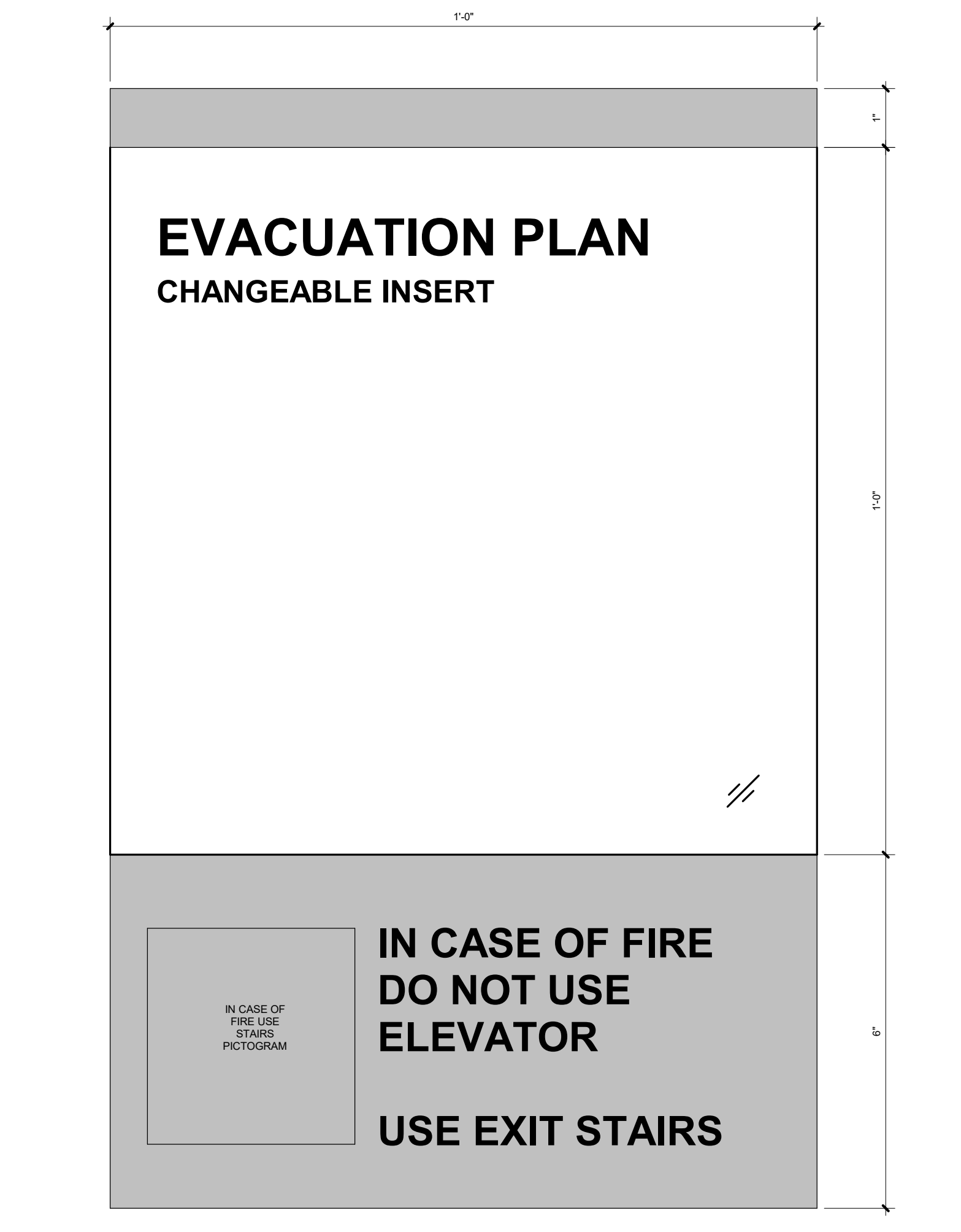
S-4 SCALE: 6" = 1'-0"
