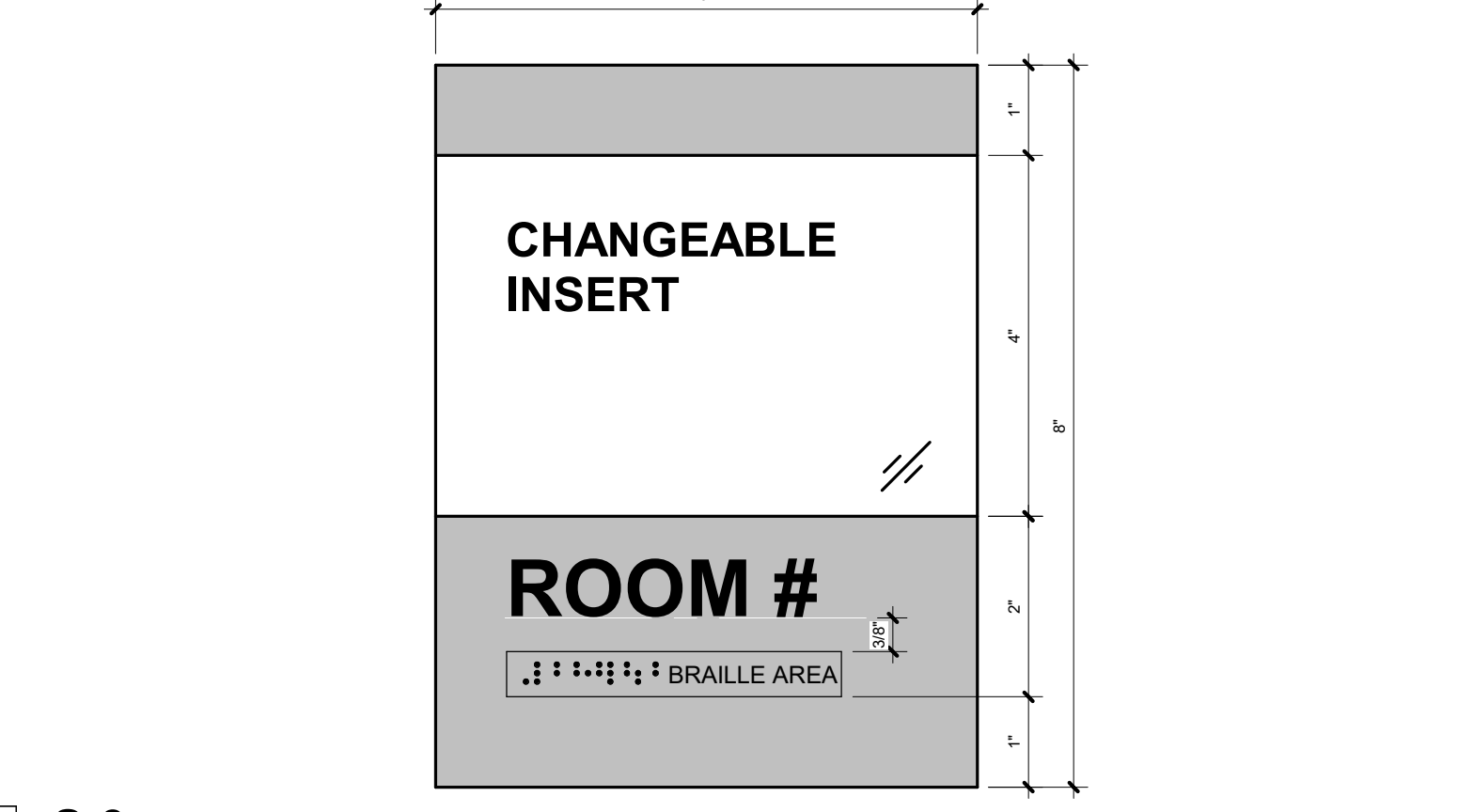
S-3 SCALE: 6" = 1'-0"
