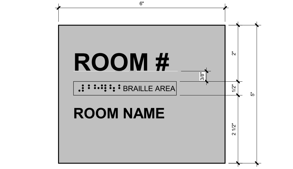
S-1 SCALE: 6" = 1'-0"
