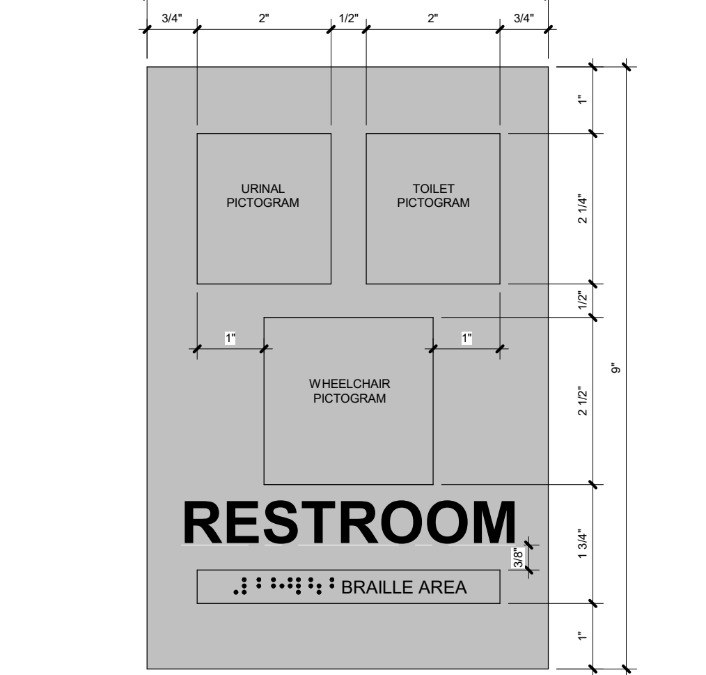
S-2B SCALE: 6" = 1'-0"
