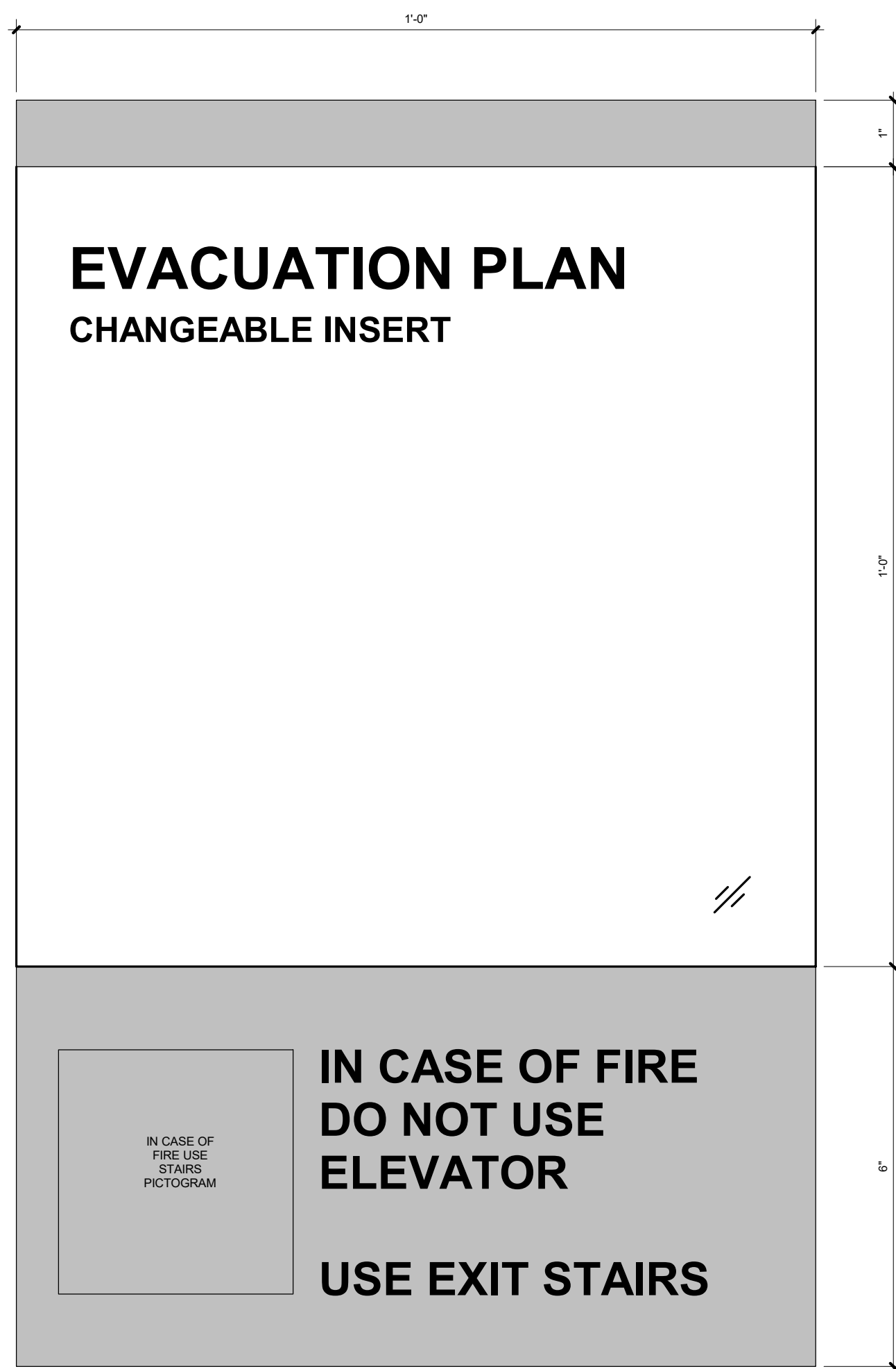
7 S-4 SCALE: 6" = 1'-0"
