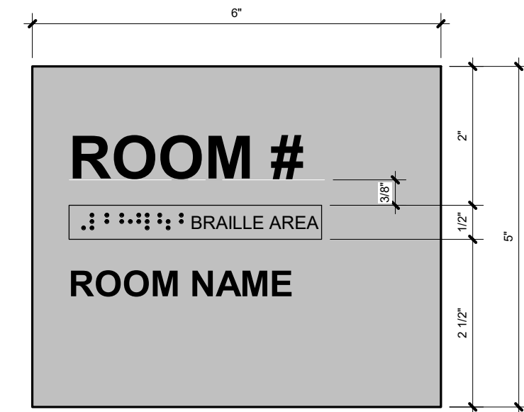
1 S-1 SCALE: 6" = 1'-0"
