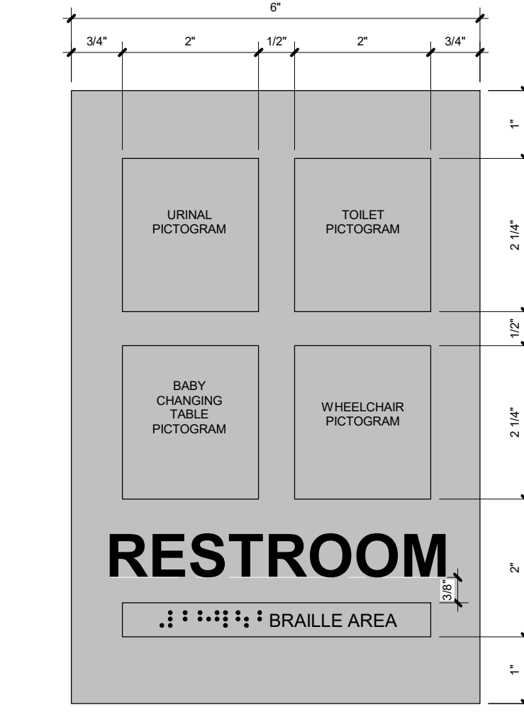
2 S-2A SCALE: 6" = 1'-0"
