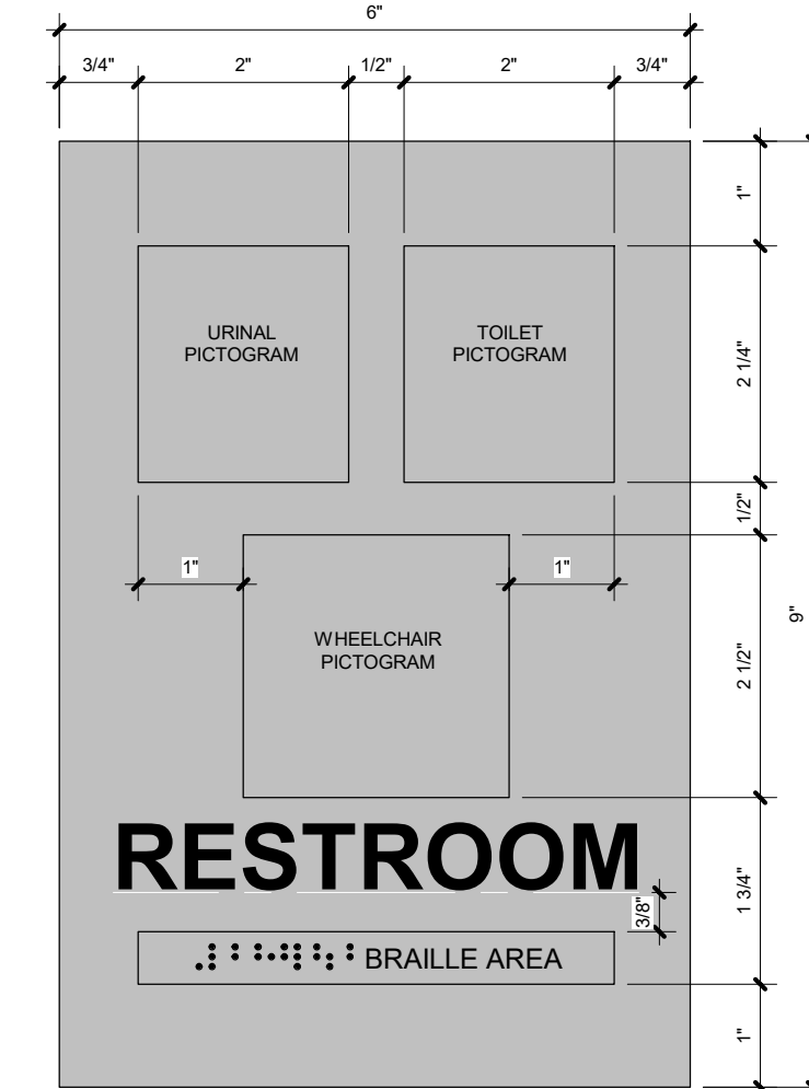
3 S-2B SCALE: 6" = 1'-0"
